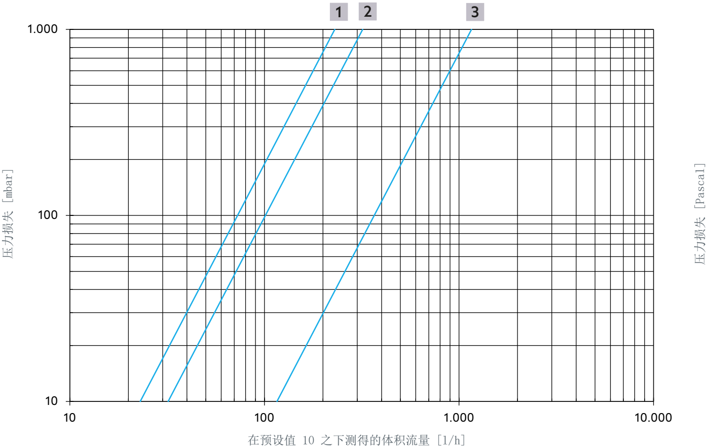
图 18: 产品编号 4202553 和 4202753 的体积流量热力调节
