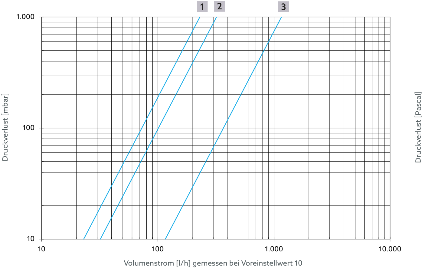
Abb. 18: Volumenstrom Thermische Regelung für Artikelnummer 4202553 und 4202753
