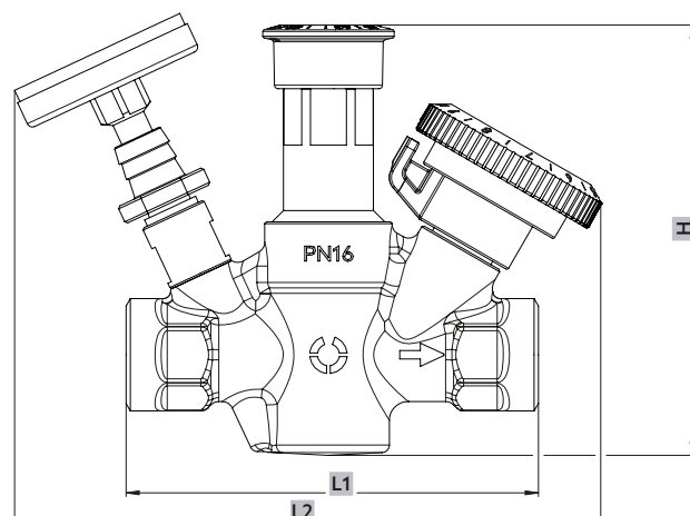
Afb. 2: Afmetingen lateraal
