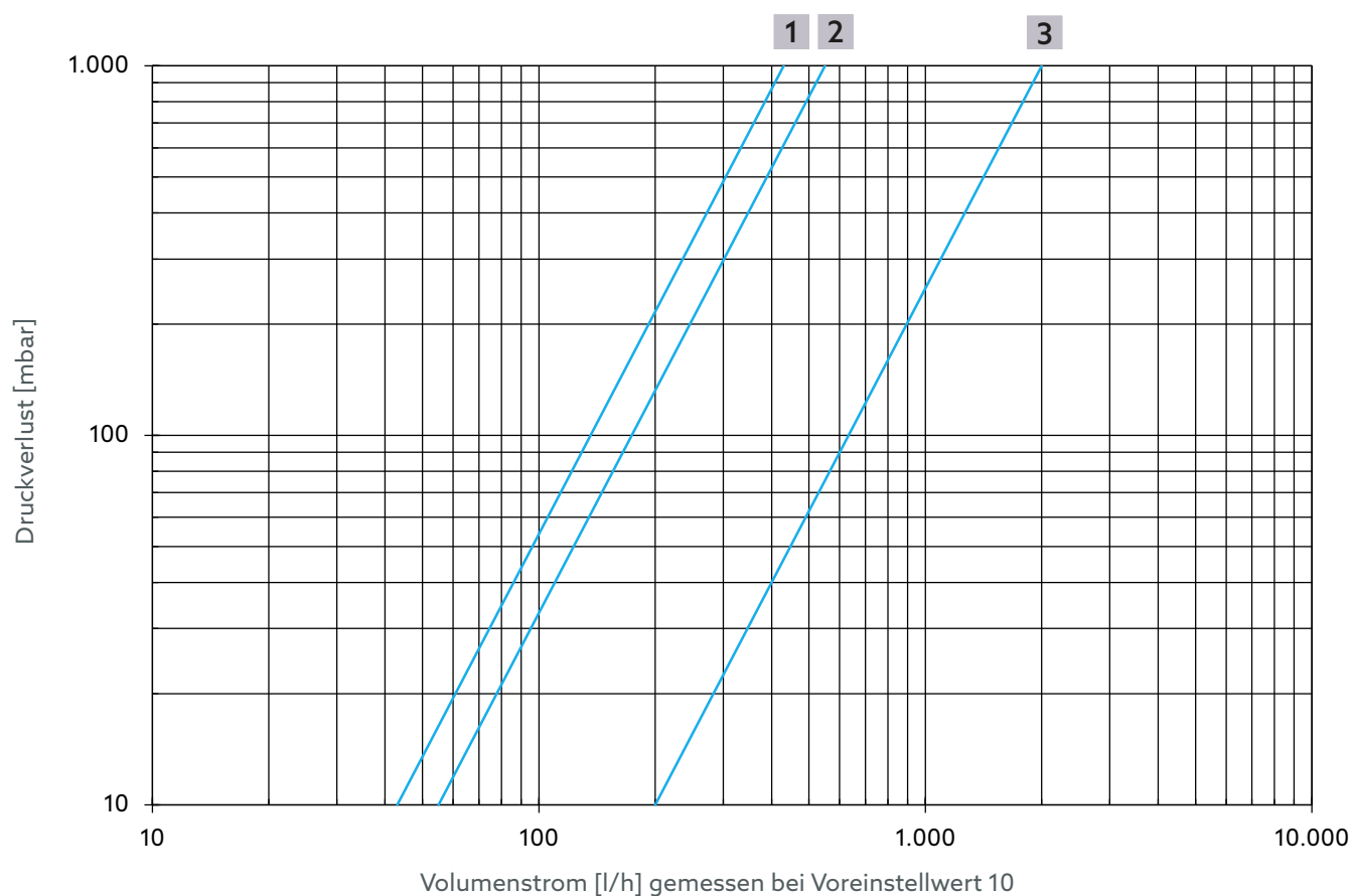
Abb. 20: Volumenstrom Thermische Regelung für Artikelnummer 4202554 und 4202754
