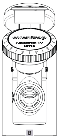
Fig. 3 - Dimensioni del lato frontale
