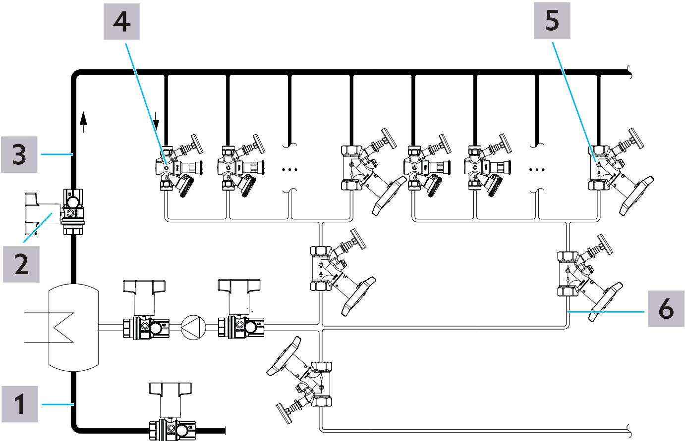
Fig. 4 - Schema dell'impianto
