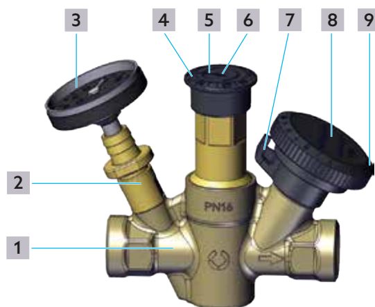
Рис. 1: Конструкция
