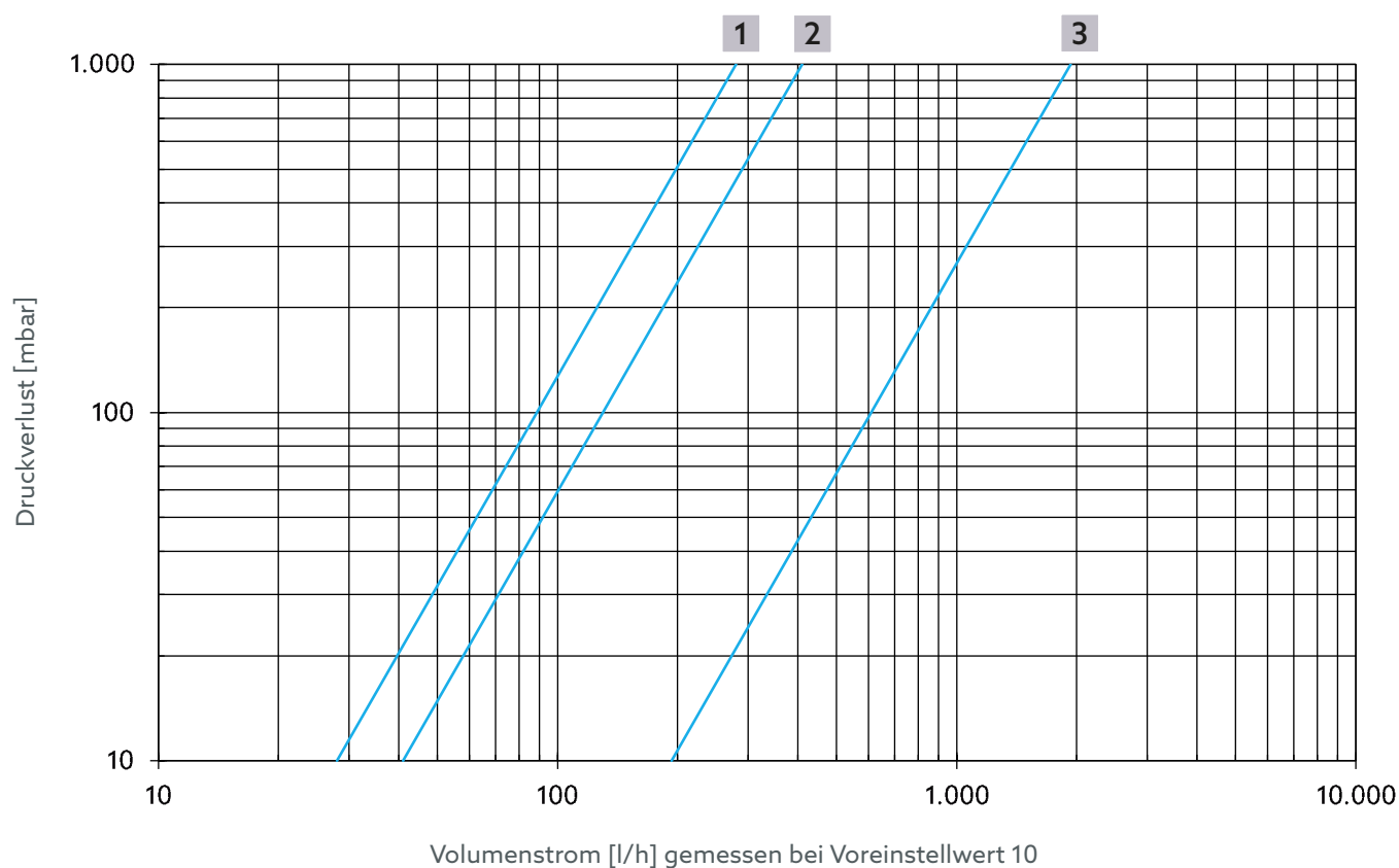
Abb. 19: Volumenstrom Thermische Regelung für Artikelnummer 4202506, 4202606, 4202706, 4202806
