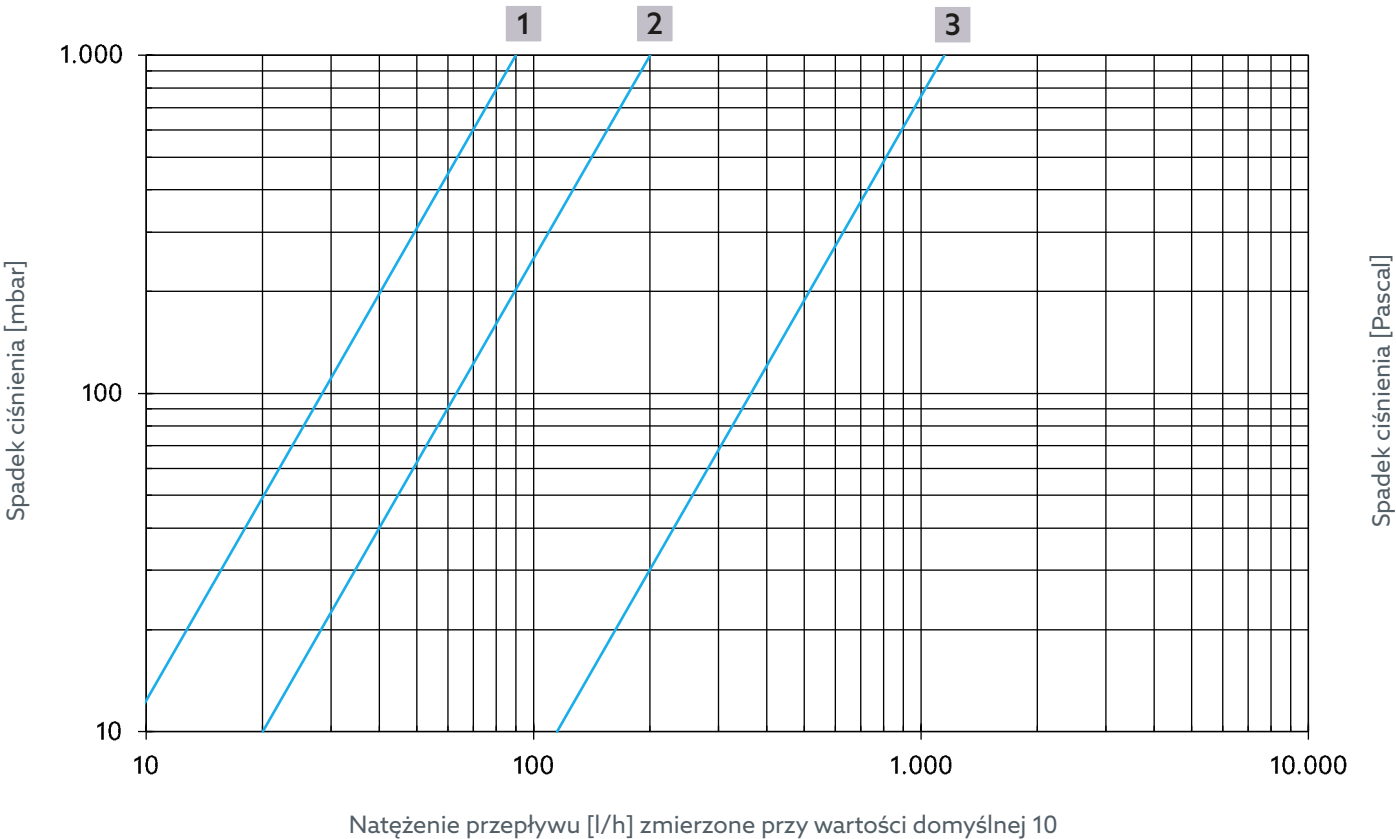
Ryc. 17: Natężenie przepływu regulacji termicznej dla artykułów numer 4202504, 4202604, 4202704, 4202804
