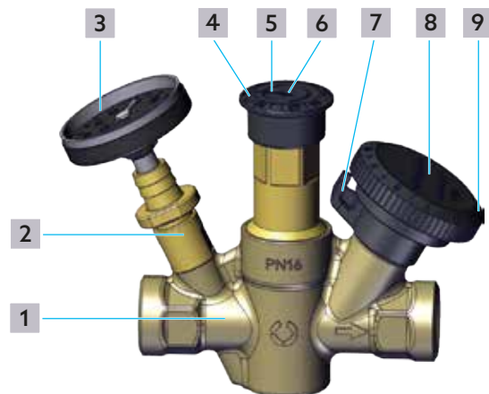
Afb. 1: Opbouw
