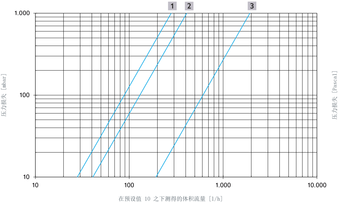
图 19: 产品编号 4202506 和 4202506, 4202606, 4202706, 4202806 的体积流量热力调节
