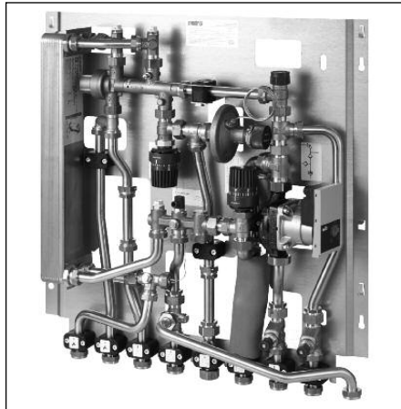
Abb. 1.1 „Regudis W-HTF“ Wohnungsstation mit Hochtemperaturkreis
