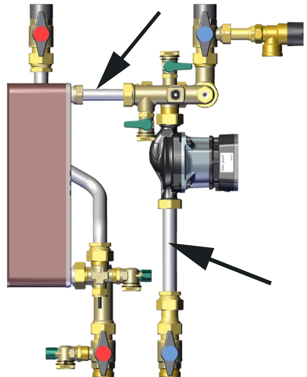
Fig. 17: Conexión equipotencial
