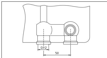
Abb. 7 Ventilgarnitur G 1/2 IG
