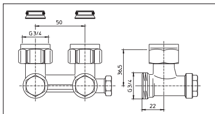
Abb. 5 Eckform, G 3/4 ÜM x G 3/4 AG
