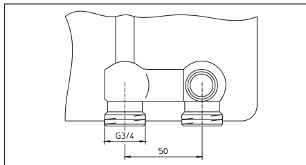
Abb. 8 Ventilgarnitur G 3/4 AG nach DIN EN 16313 (Eurokonus)
