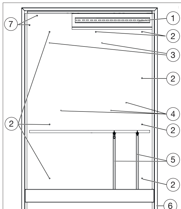
Fig. 2: Construction coffret pour pose en applique 1344698 et 1344699
