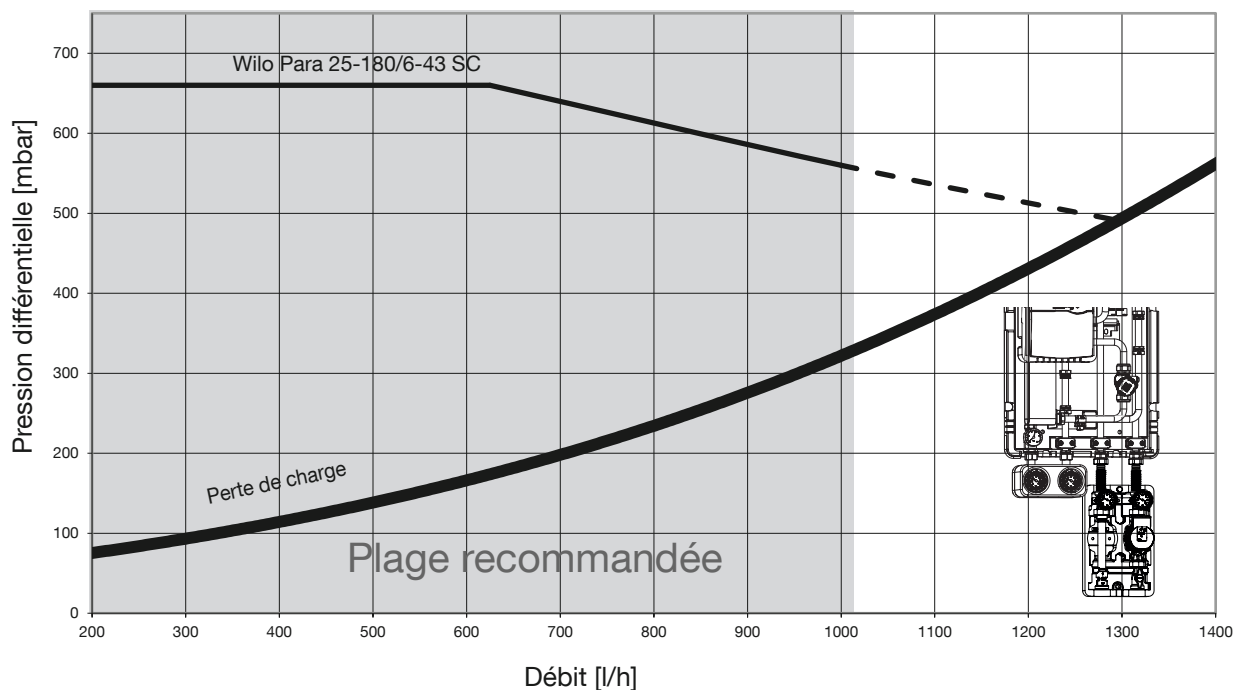
Fig. 5: Perte de charge circuit secondaire Regudis H-M
