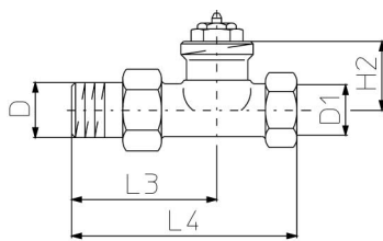
Durchgangsgehäuse
