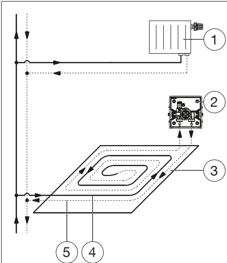
Abb. 10: Anschluss
