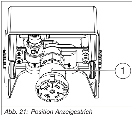
Abb. 21: Position Anzeigestrich
