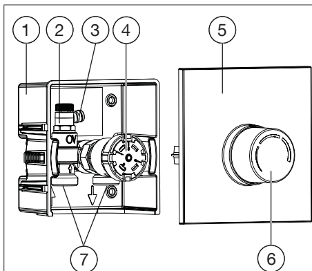
Abb. 2: Aufbau Unibox RTL
