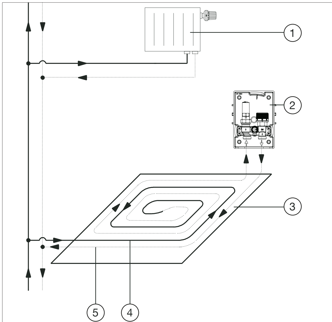
Abb. 1: Anschluss
