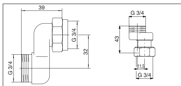
Dimensioni del raccordo a S
