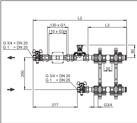
Abb. 4.2 Beispiel: Wärmemengenzähler-Anschluss-Set 1, Durchgangsform, und „Multidis SH“ Edelstahl-Verteiler für Heizkörperanbindung, Baulängen
