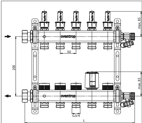
Abb. 4: Maße
