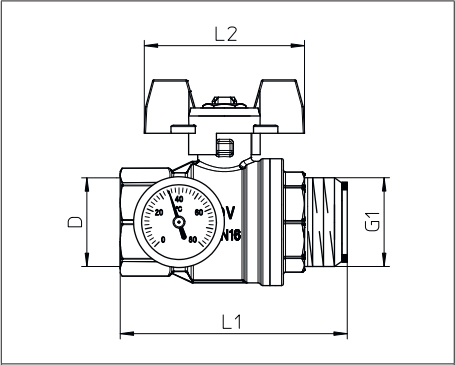
Abb. 5: Maße Kugelhahn
