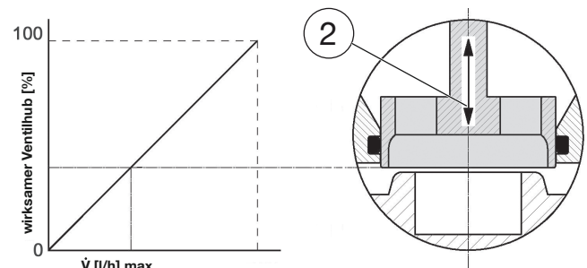
Abb. 5: Lineare Kennlinie der Reguliereinheit
