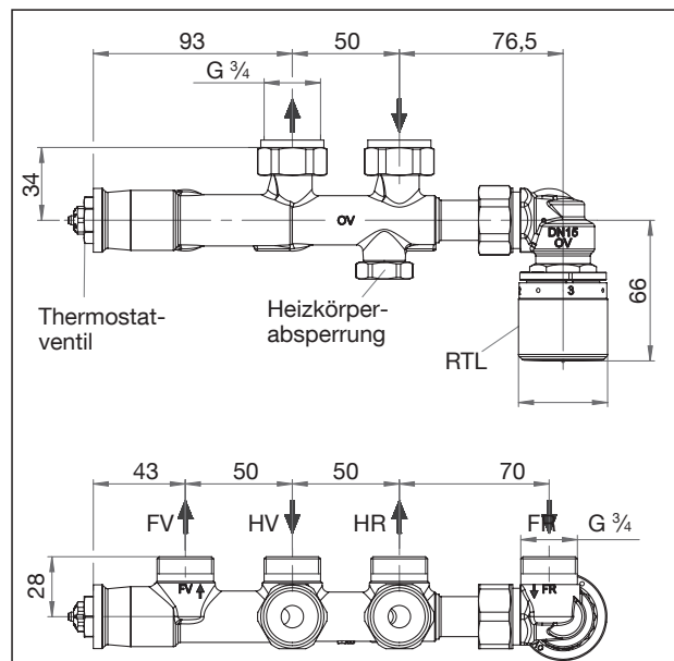
Abmessungen Armatur
