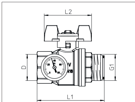
Рис.6: Размеры шарового крана
