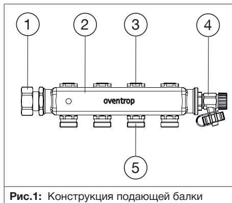
Рис.1: Конструкция подающей балки
