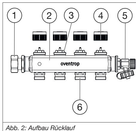
Abb. 2: Aufbau Rücklauf
