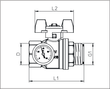
Abb. 6: Maße Kugelhahn
