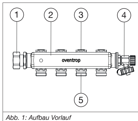
Abb. 1: Aufbau Vorlauf
