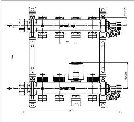
Abb. 5: Maße
