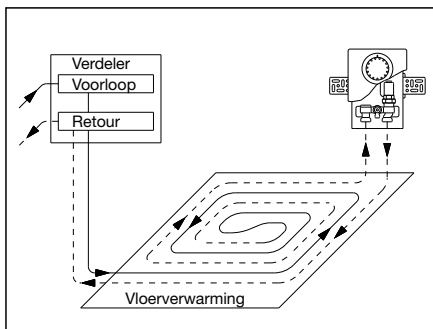
Inbouwplan
