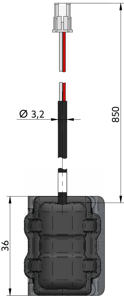
Fig. 2: Dimensions
