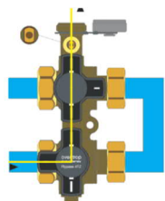
Entleeren und entlüften der Anlage- und Geräteseite, spülen der Anlage
