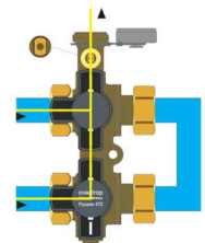
Befüllen und entlüften der Anlage
