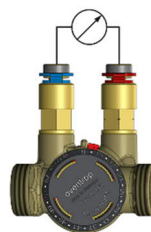
Differenzdruckmessung über das Cocon QTZ.
