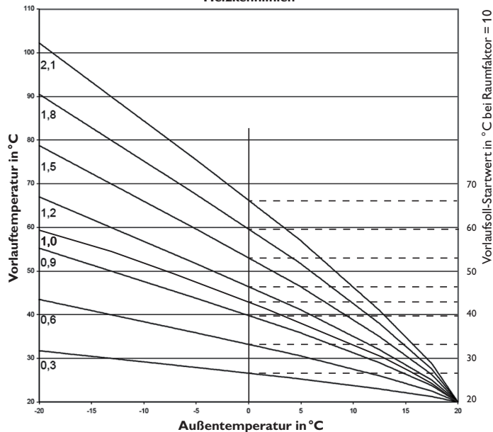
Heizkennlinien
