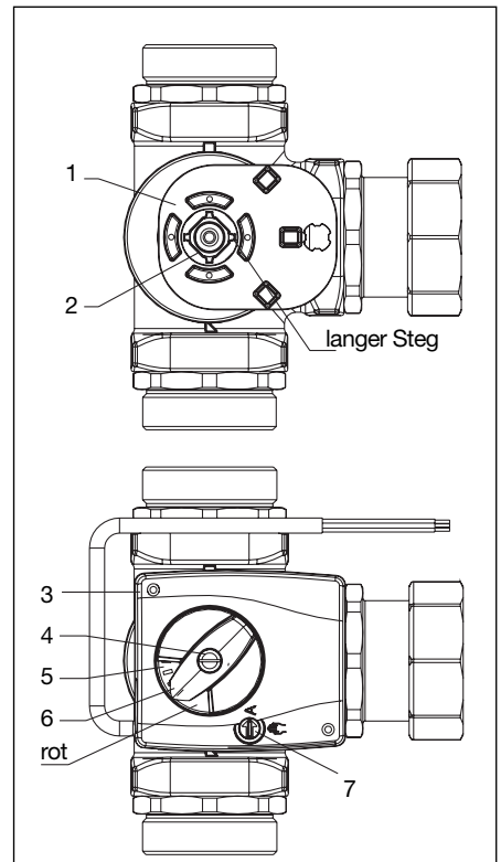
Abb. 5.2 Montage 3-Wege-Mischhahn DN 40 / DN 50
