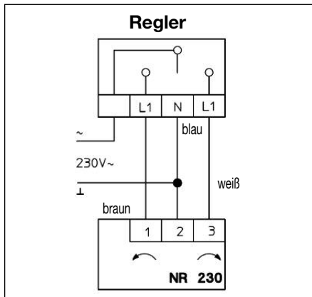
Abb. 5.1 Anschluss-Schema Dreipunktsteuerung
