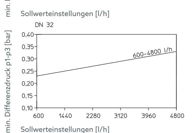
Abb. 13: Mindest-Differenzdrücke
