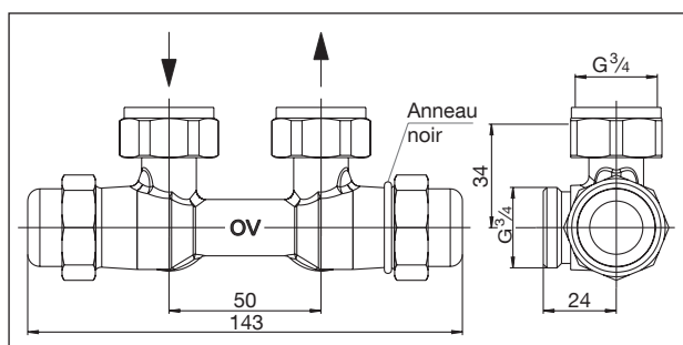
Corps de robinet équerre
