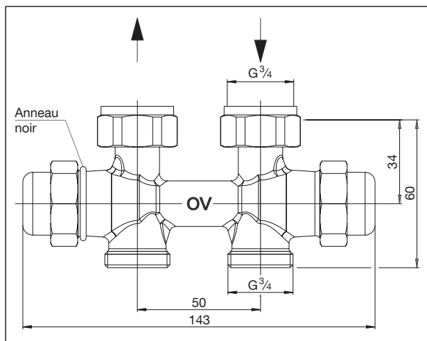
Corps de robinet droit
