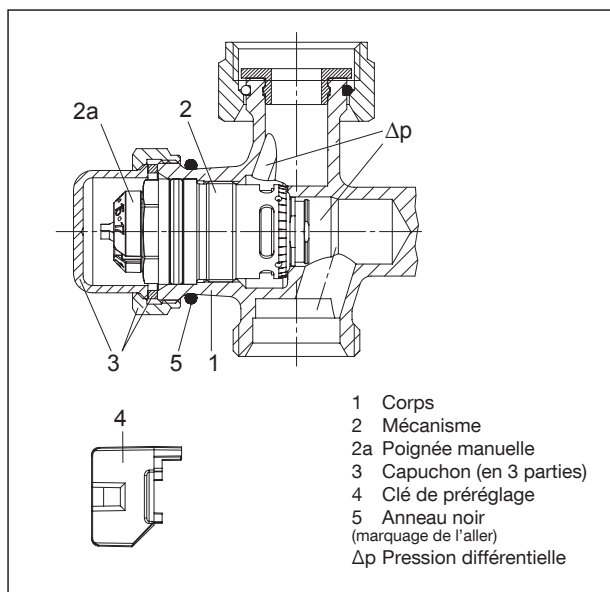
Configuration du régulateur de débit
