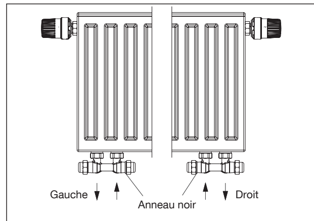
Affectation des raccords des modèles équerres pour raccordement à gauche ou à droite
