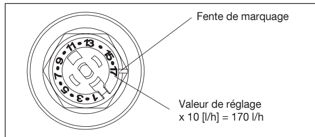
Réglage du débit
