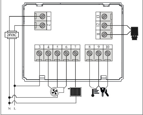
Abb. 5: Anschlussschema 1152064
