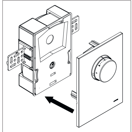
Abb. 11: Abdeckplatte mit Handrad aufsetzen
