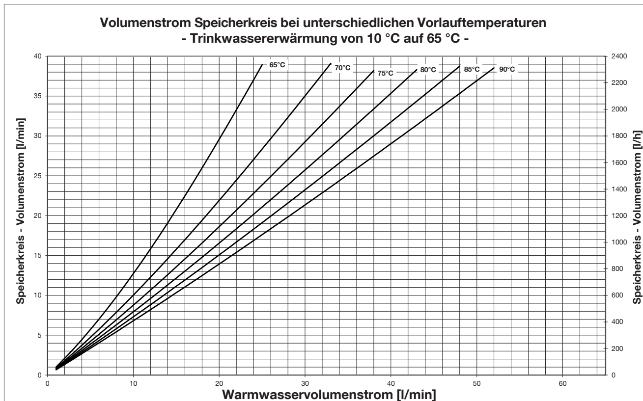
Fig. 14: Débit dans le circuit ballon d'eau chaude - Réchauffage de l'eau potable à 65 °C
