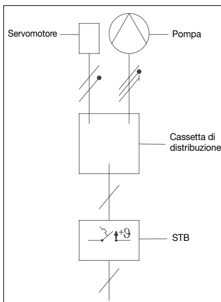
Fig. 4.1 Schema cablaggi
