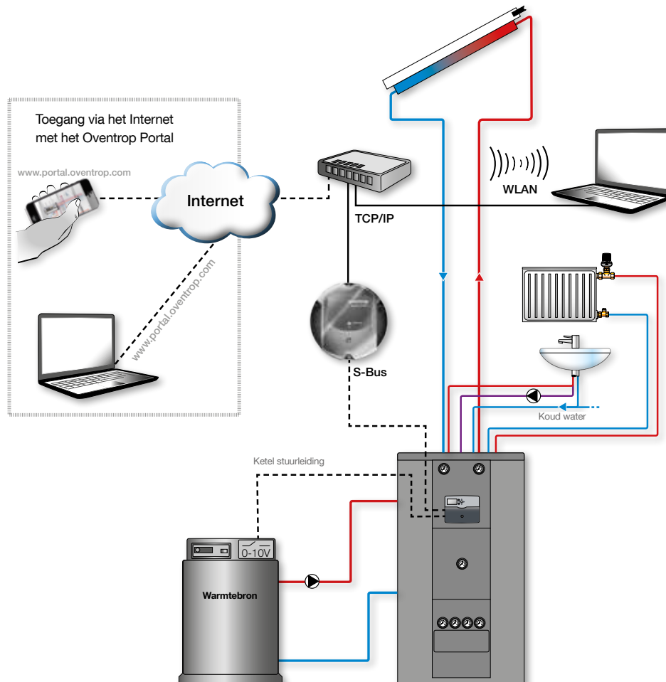
Regucor WHS energieopslagsysteem voor zonneverwarming, tapwater en verwarming
