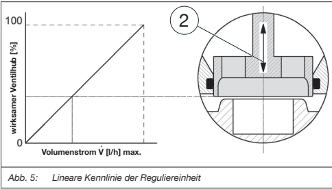
Abb. 5: Lineare Kennlinie der Reguliereinheit
