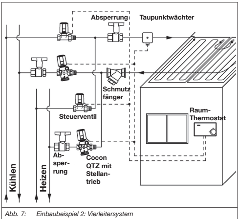
Abb. 7: Einbaubeispiel 2: Vielleitersystem
