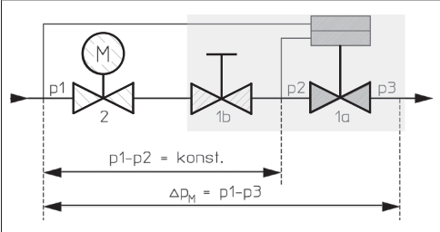
Abb. 3: Funktionsprinzip „Cocon QTZ“, PN25
