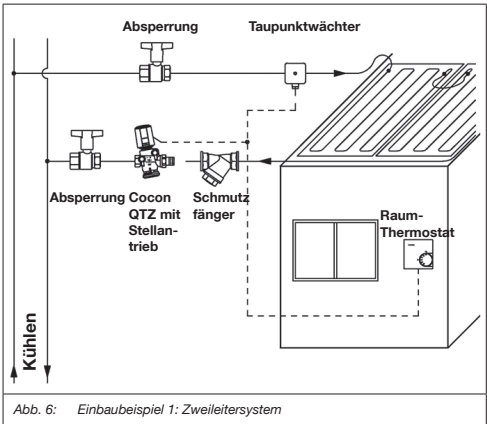
Abb. 6: Einbaubeispiel 1: Zweileitersystem
