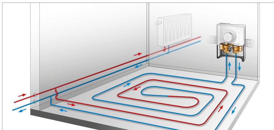
„Unibox TQ“ Einsatzbeispiel inkl. Flächenheizung
