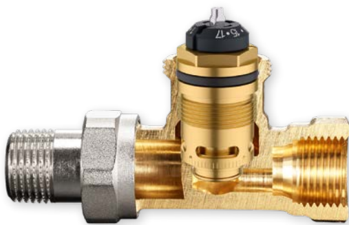
Querschnitt „AQ“ Durchgangsventil
