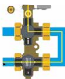
Vullen en spoelen van de installatie
