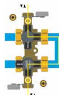
Bijvullen, ontluichten en spoelen van de installatie, met een tweede kogelkraan voor vullen/aftappen
