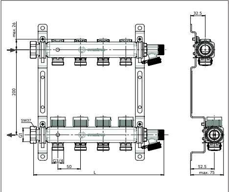
Fig. 5: Maße
