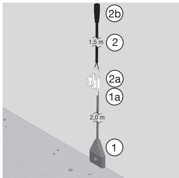
Abb. 37: Anschluss Feuchtefühler/Sensorkabel an Regler
