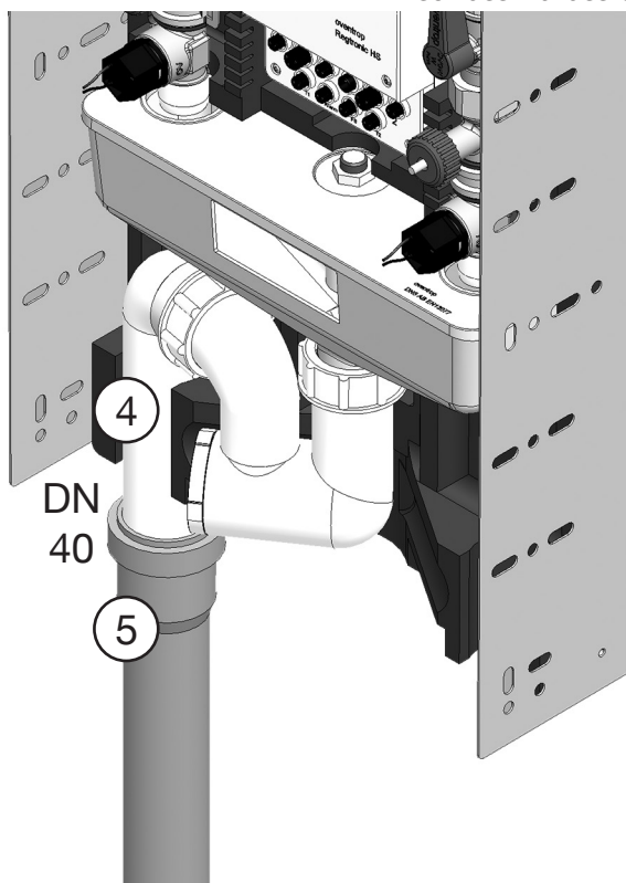
Abb. 32: Anschluss Abflussrohr
