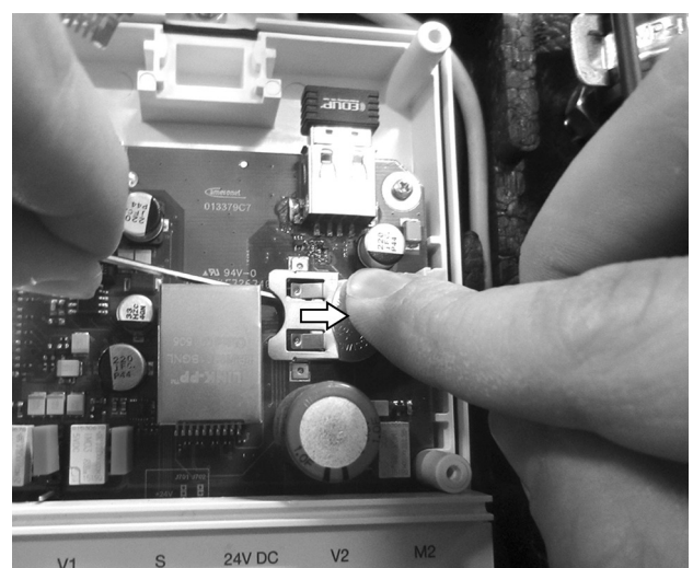
Abb. 130: Leere Batterie nach rechts herausdrücken
