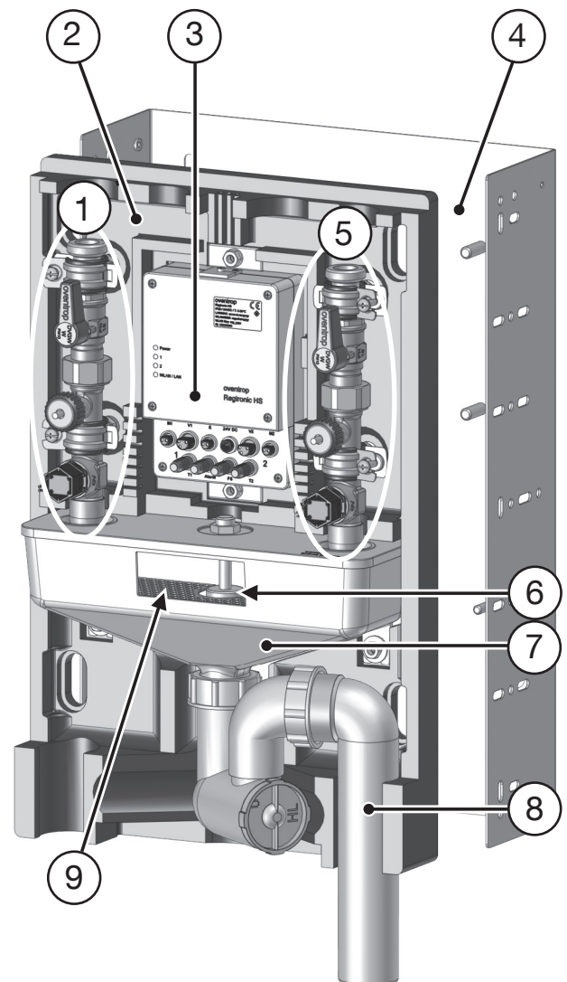
Spülstation „Duo“ (2-Strang Trinkwasser)
