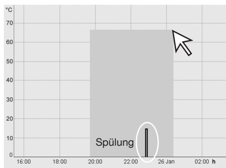
Abb. 109: Temperaturveränderung nach eingeleiteter Spülung (Detailansicht)
