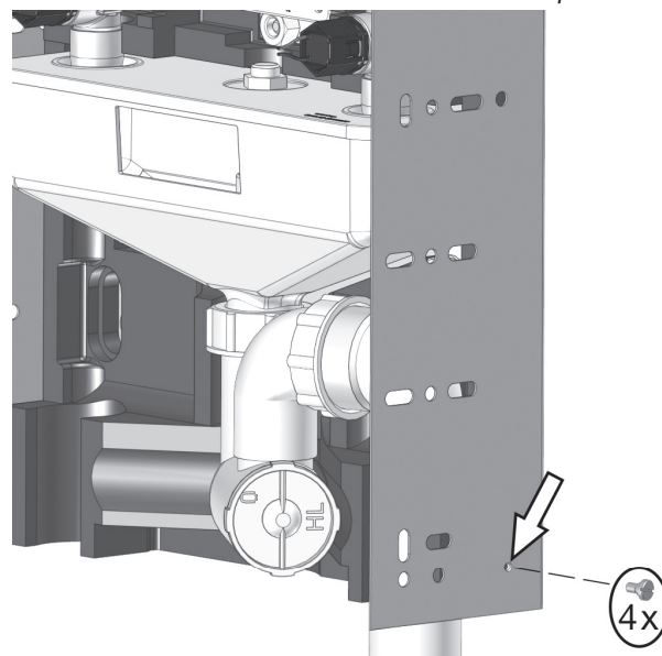
Abb. 28: Schrauben für Aufnahme Aufputzhaube
