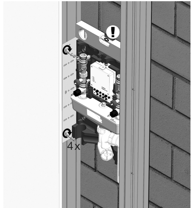
Abb. 29: Montage Spülstation in Ständerwerk
