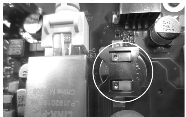
Abb. 129: Speicherbatterie in Halterung
