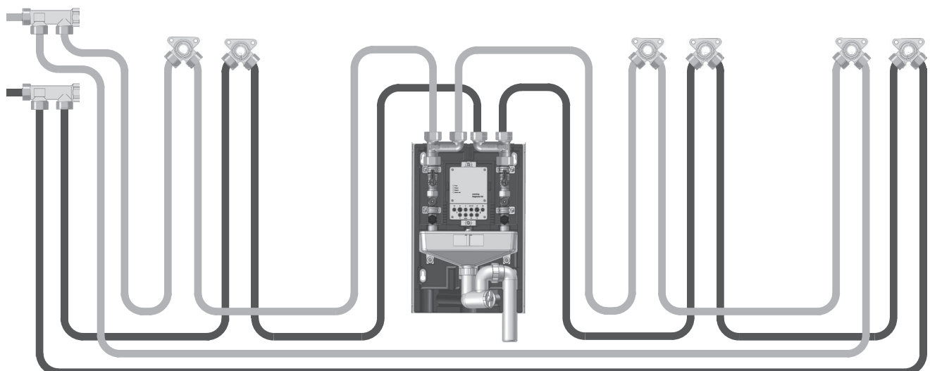
Spülstation „Regudrain Duo“ (2-Strang) an Ringleitung (Beispiel)
