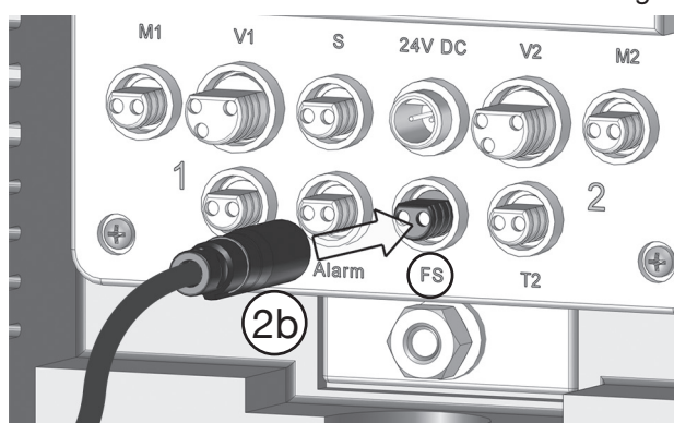
Abb. 37: Anschluss Feuchtefühler/Sensorkabel an Regler
