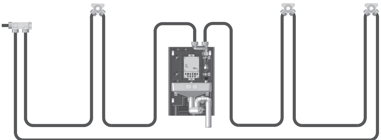
Spülstation „Regudrain Uno“ (1-Strang) an Ringleitung (Beispiel)
