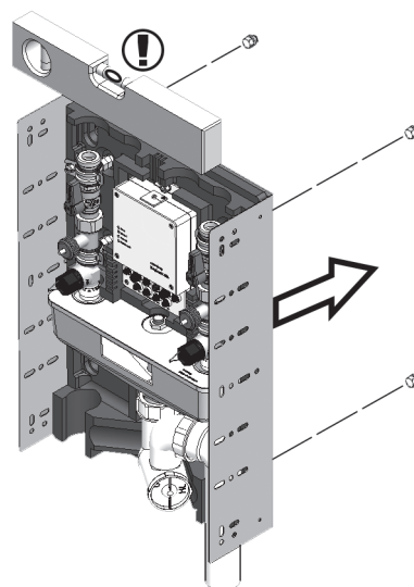
Abb. 27: Siphon-Rohr aus Unterschale lösen
