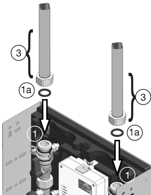
Abb. 31: Montage „Regudrain Duo“ in Reihenleitung
