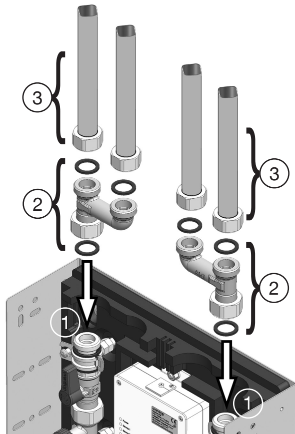
Abb. 30: Montage „Regudrain Duo“ in Ringleitung
