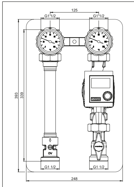
Abb. 5 „Regumat S-180“ DN25 mit Pumpenkugelhahn (kurze Bauform)
