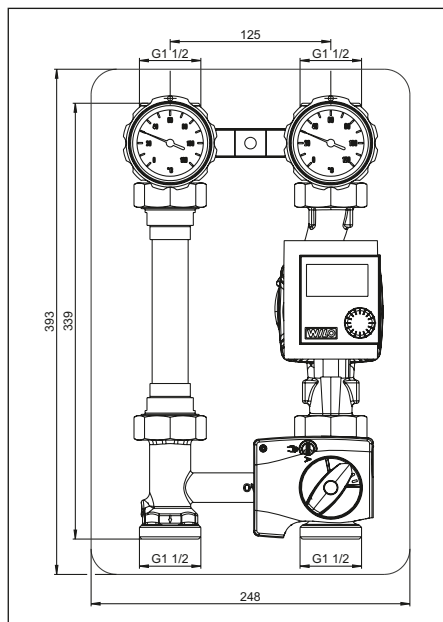
Abb. 6 „Regumat M3-180“ DN25 mit Pumpenkugelhahn (kurze Bauform)
