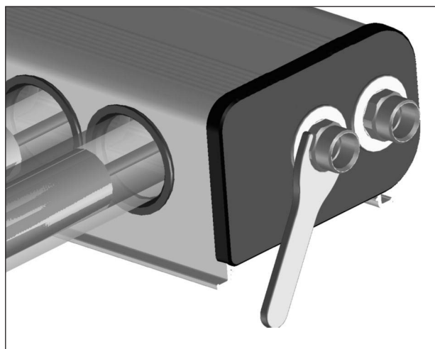
Abb. 29: Kollektoran- schlüsse gegenhalten
