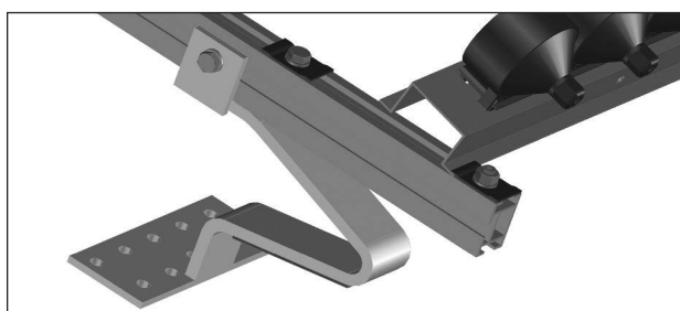
Fig. 11: Positionner le rail équerre dans le rail de montage
