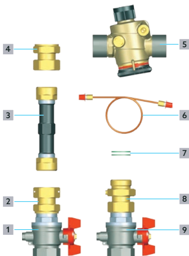
Abb. 2: Aufbau Durchgangsausführung
