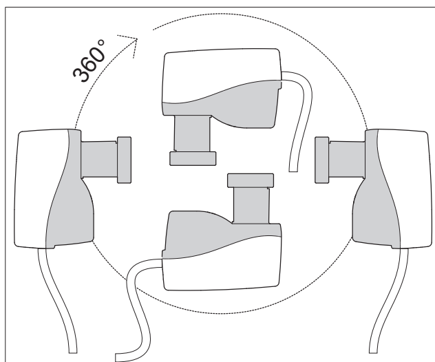
Abb. 3: Einbaulage
