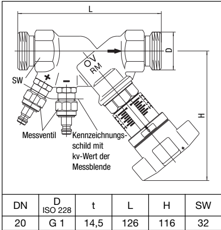
Abb. 4.1 Abmessungen „Hydrocontrol STR“ mit Klemmringanschluss
