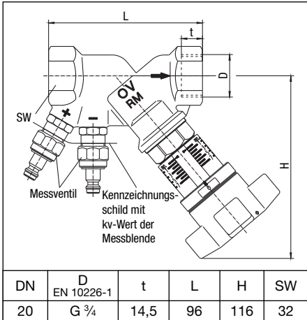
Abb. 4.2 Abmessungen „Hydrocontrol STR“ mit Innengewinde
