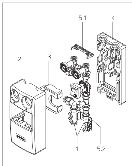
Abb. 6.1 „Regumat“-Pufferspeicher-Anschlussgruppe
