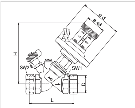
Illustr. 3: Régulateur 10646/48 04-16 filetage mâle et écrous d'accouplement des deux côtés
