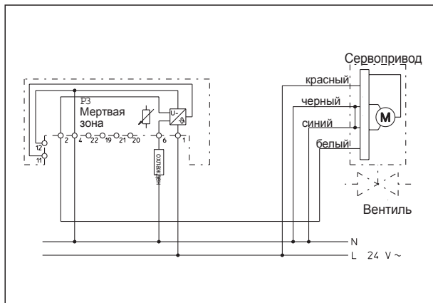
Схема переключения
