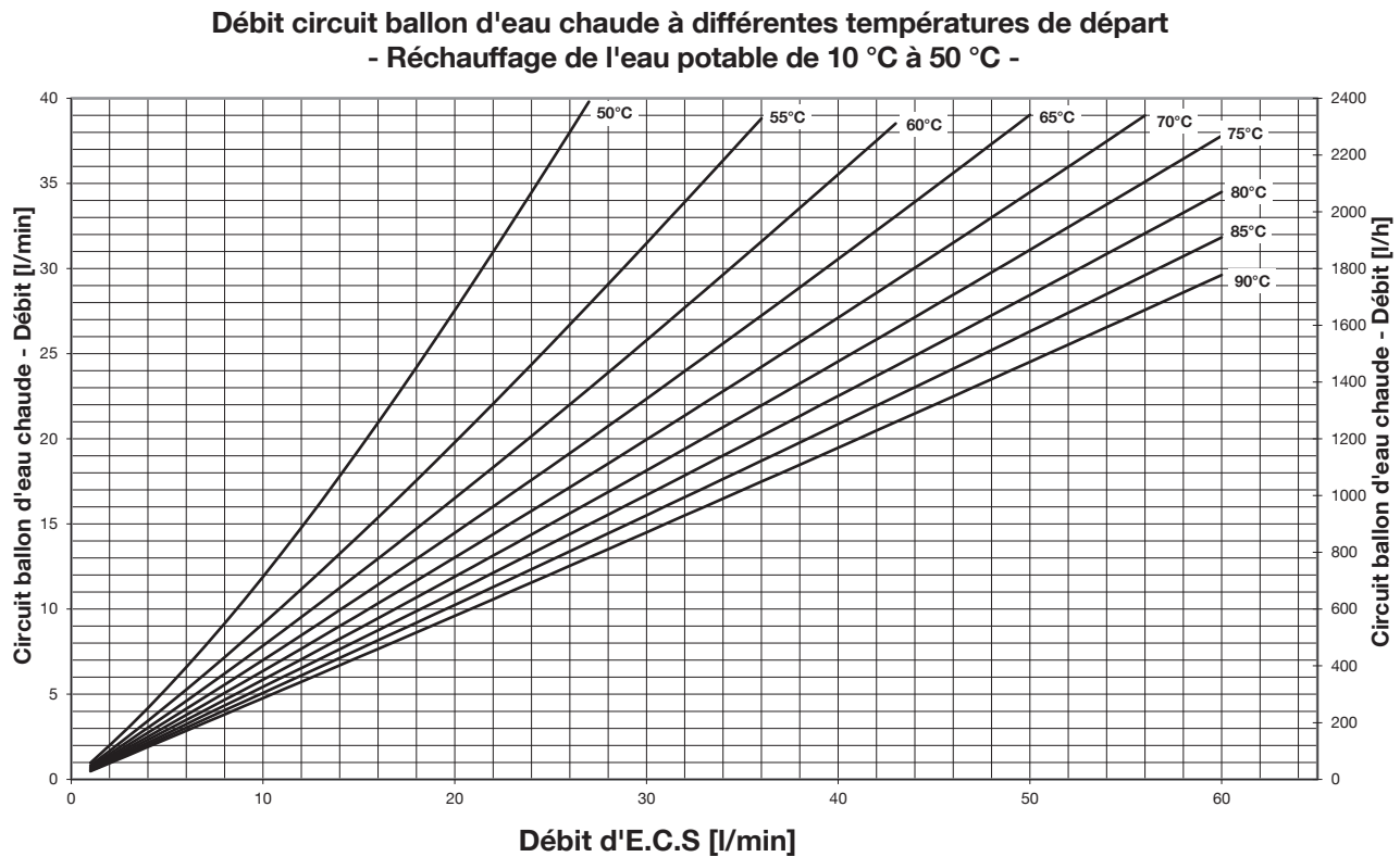
Fig. 41: Débit du circuit ballon d'eau chaude - Réchauffage de l'eau potable à 50 °C
