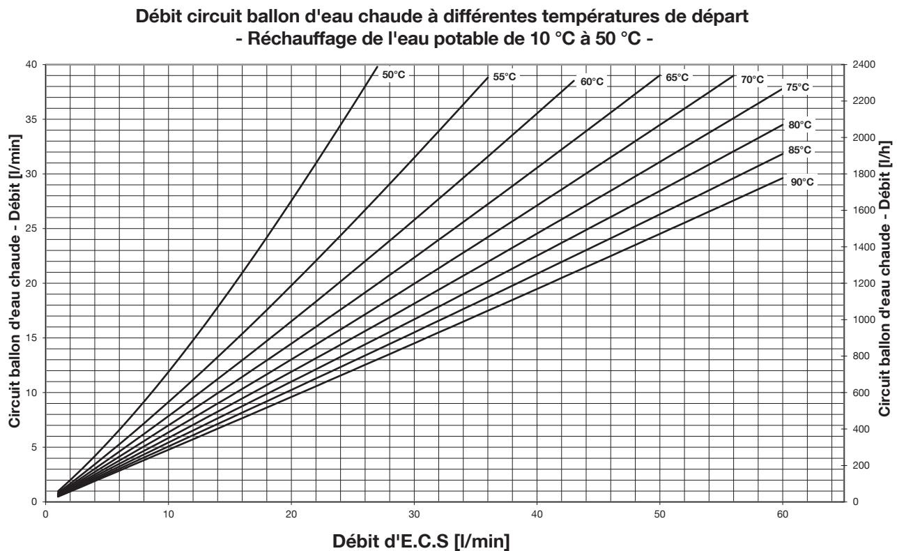
Fig. 42: Température de retour du circuit ballon d'eau chaude - Réchauffage de l'eau potable à 50 °C
