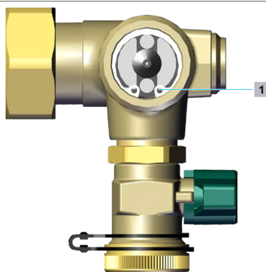
Fig. 33: Circlip
