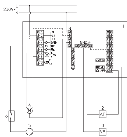
Abb. 5: Anschlussplan für witterungsgeführte Regelung
