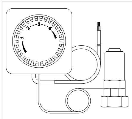
Thermostat mit Fernverstellung und Temperaturabsenkung
