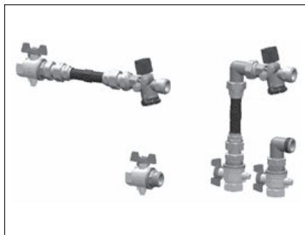
Abb. 1 Wärmemengenzähler-Anschluss-Set, Durchgangs- und Eckausführung
