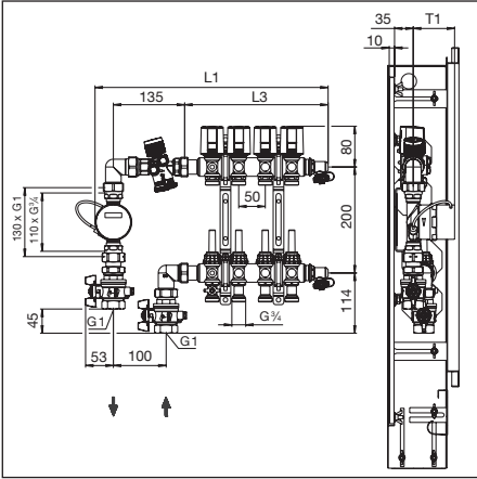
Fig. 2 Exemple : Jeu de raccordement pour compteurs de calories, modèle équerre et distributeur/collecteur « Multidis SF » pour installations de surfaces chauffantes, longueurs et profondeur
