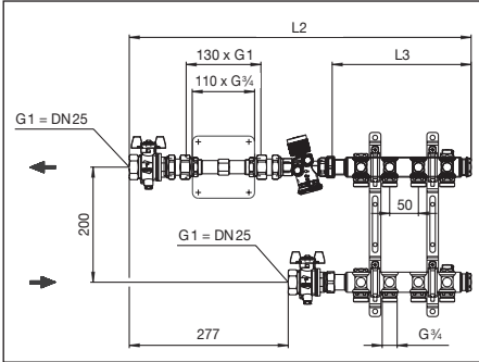
Fig. 3 Jeu de raccordement pour compteurs de calories, modèle droit et distributeur/collecteur en acier inoxydable «Multidis SH» pour le raccordement de radiateurs, longueurs
