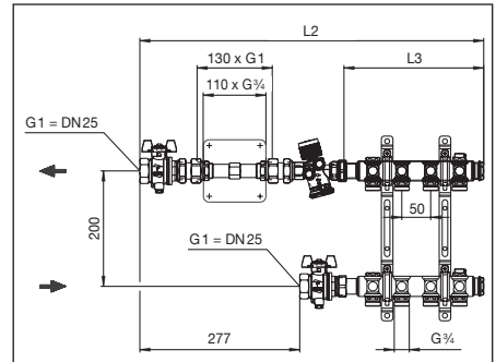
Abb. 3 Wärmemengenzähler-Anschluss-Set, Durchgangsform, und „Multidis SH“ Edelstahl-Verteiler für Heizkörperanbindung, Baulängen
