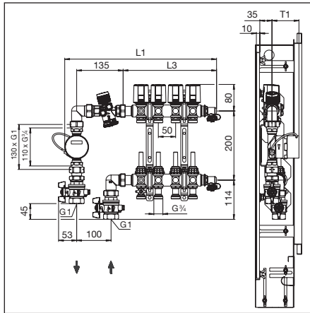
Abb. 2 Beispiel: Wärmemengenzähler-Anschluss-Set, Eckform und „Multidis SF“ Edelstahl-Verteiler für Flächenheizung, Baulängen und Bautiefe
