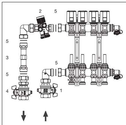
Abb. 4: Wärmemengenzähler-Anschluss-Set , Eckform, Lieferumfang und Anordnung der Komponenten bei Linksanschluss.
