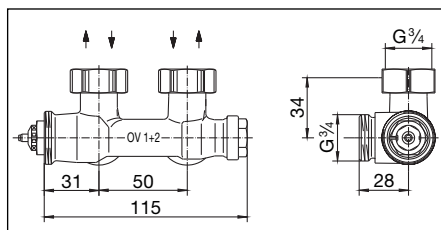
Fig. 6 Modèle équerre
