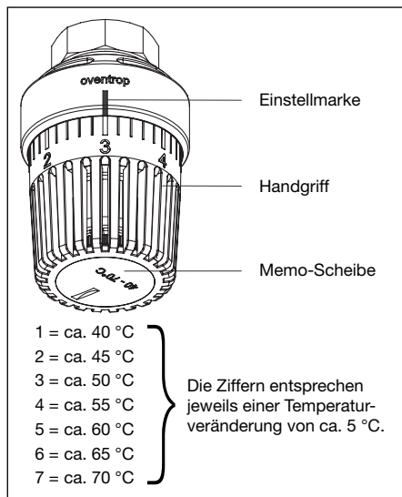
Abb. 7.3 Einstellung Trinkwassertemperatur
