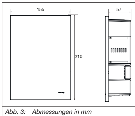
Abb. 3: Abmessungen in mm
