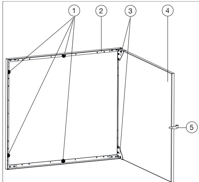
Abb. 1: Aufbau Revisionsrahmen
