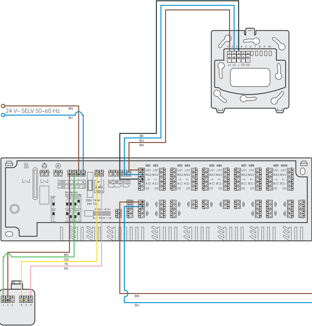
Taupunktwächter 24 V 1141951 Dew point monitor
