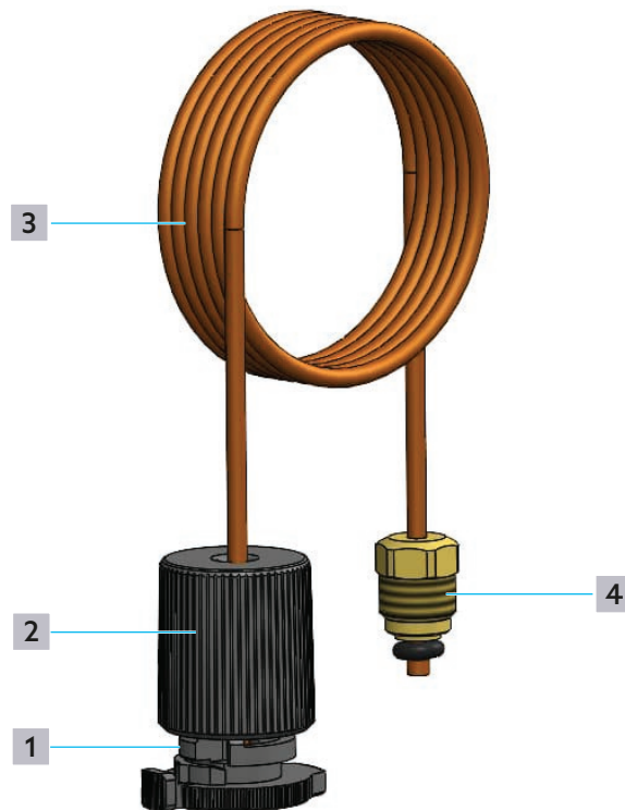
Obr. 4: Montáž impulzního vedení
